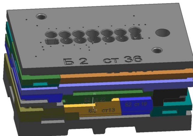
Габаритные размеры: 800 x 405 x 335 мм Масса отливки: около 150 кг
