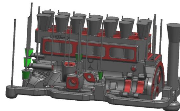
Габаритные размеры: 1000 x 575 x 520 мм Масса отливки: около 280 кг
